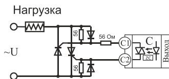
Подключение внешних тириستоров к выходу “С”
